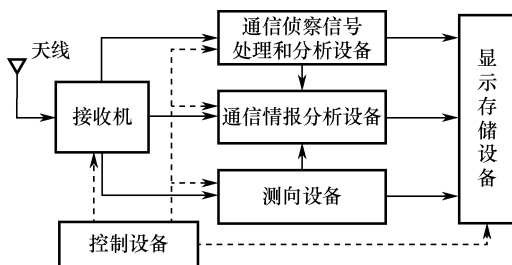
图 1-1 通信对抗侦察设备原理框图
