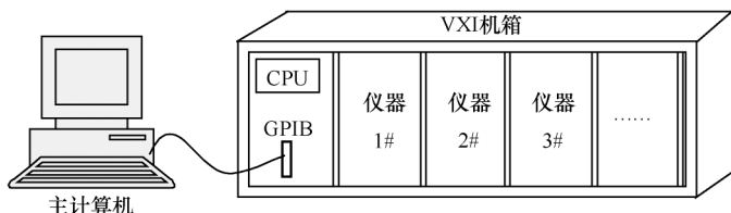
图 1.6 典型的基于 VXI 模块化仪器的个人仪器测试系统
