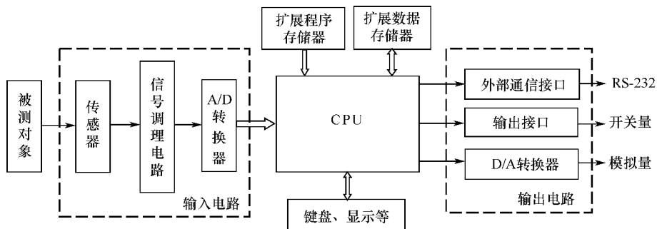
图 1.4 内嵌微处理器测试系统的结构
