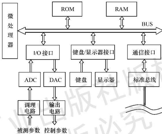
图 1.1 智能仪器的典型结构
