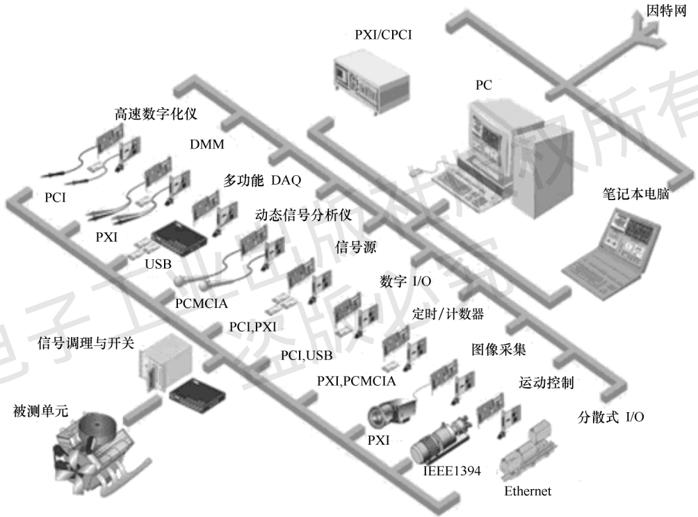
图 1.3 虚拟仪器的组成结构
