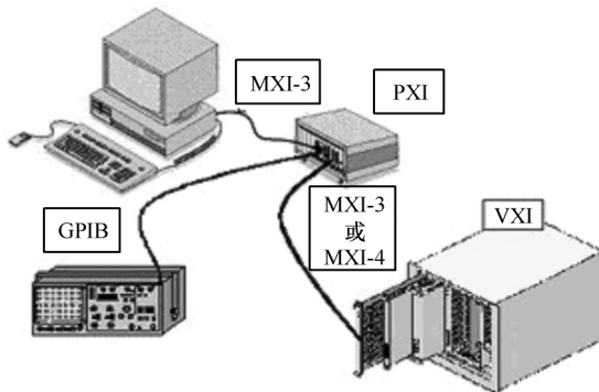
图 1.2 典型的自动测试系统组成结构
